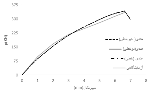
شکل ۹: مقایسه نمودارهای بار-تغییر مکان محاسباتی تیر OA1 نمودار آزمایشگاهی
