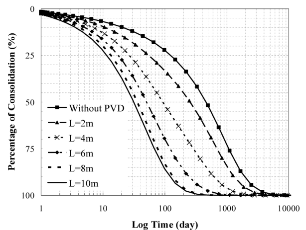
شکل ۲: نتایج درصد تحکیم در طول زمان برای طول‌های مختلف PVD
