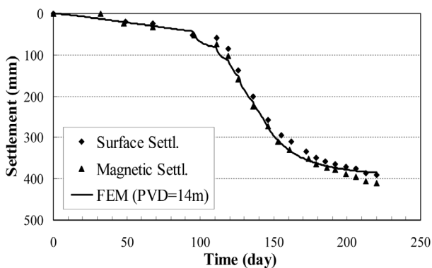
شکل ۱۰: نمودار نشست سطحی خاک در طول زمان برای ابزارها و مدل عددی تقارن محوری
