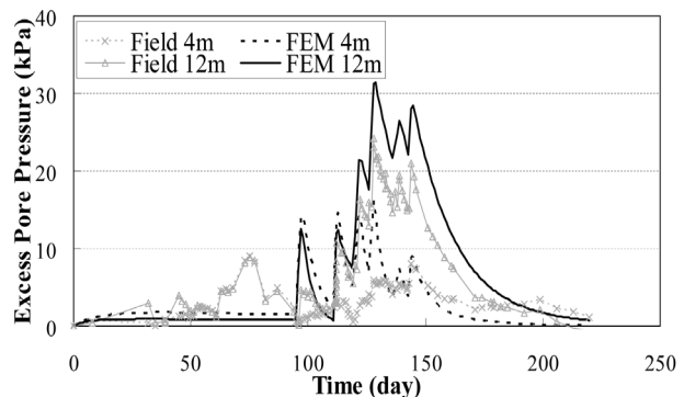
شکل ۱۲: تغییرات اضافه فشار آب حفره‌ای در طول زمان و در اعماق ۴ و ۱۲ متری حاصل از مدل عددی و پیزومتر تار لرزان (PVD = متر)
