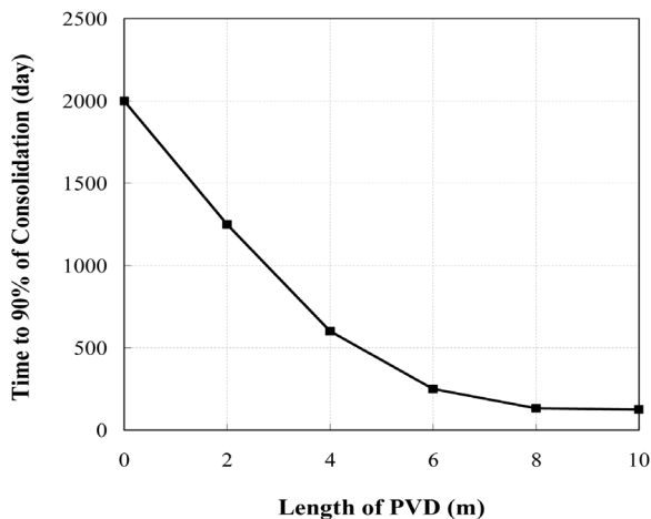
شکل ۴: زمان رسیدن به ۹۰ درصد تحکیم بر حسب طول‌های مختلف PVD
