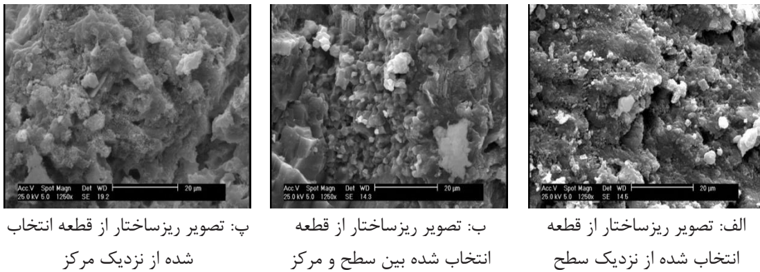
شکل ۱۴. تصاویر ریزساختار از نمونه بتنی حاوی افزودنی.
