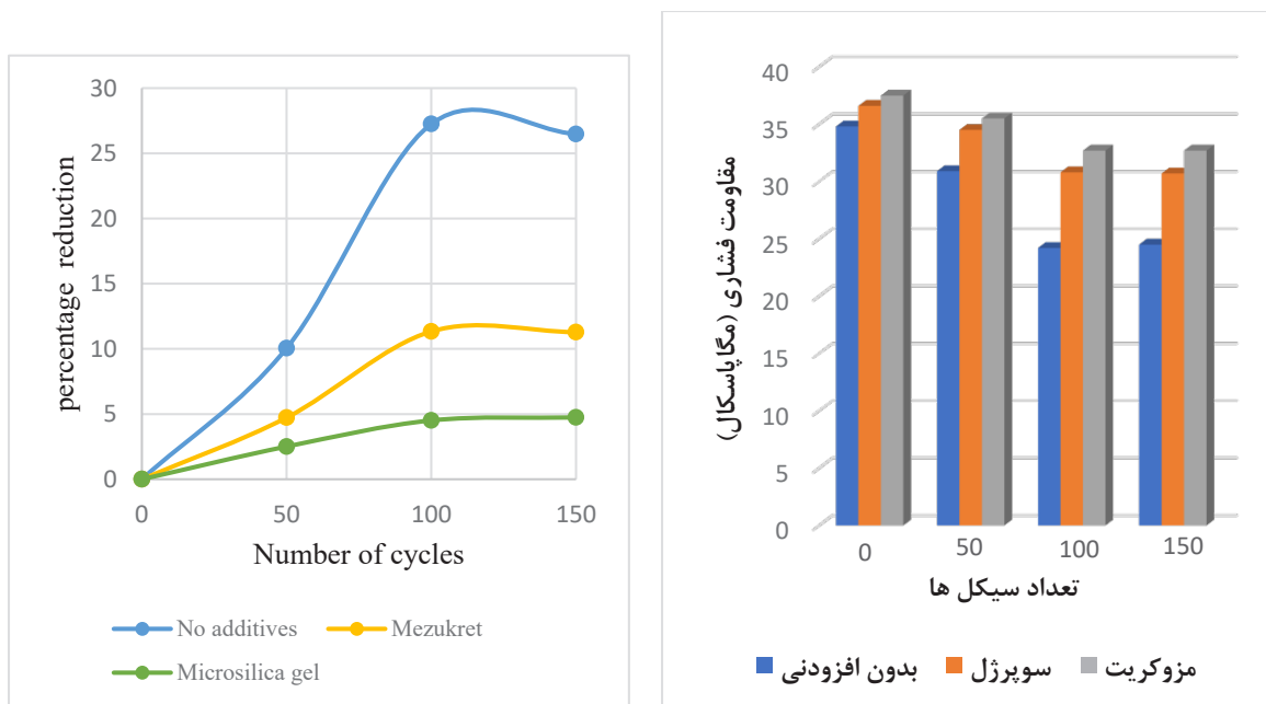
(ب) درصد کلی کاهش مقاومت فشاری در سیکل‌های مختلف
