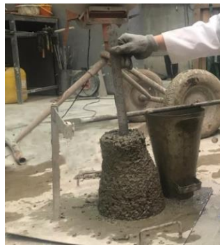
(ج) اندازه‌گیری اسلامپ (c) measuring slump
