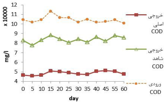
شکل ۲: نمودار غلظت ورودی و خروجی COD در تالاب شاهد و اصلی
