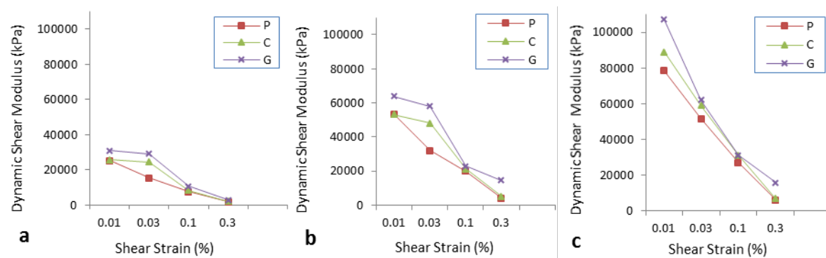
شکل ۹. مدول برشی دینامیکی - کرنش برشی برای خاک طبیعی (P)، خاک-سیمان (C)، خاک-ژئوپلیمر (G) با ۲۵٪ لای (a) فشار همه جانبه ۵۰ kPa (b) فشار همه جانبه ۱۰۰ kPa (c) فشار همه جانبه ۱۵۰ kPa
