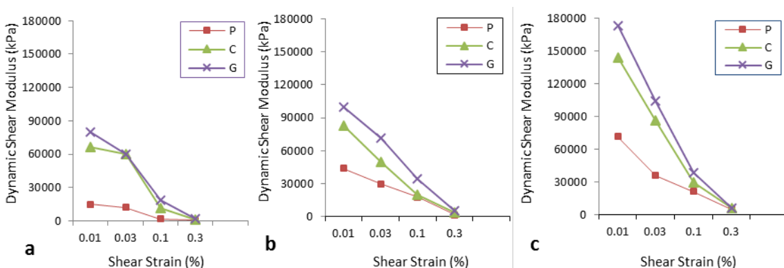
شکل ۱۰. مدول برشی دینامیکی - کرنش برشی برای خاک طبیعی (P)، خاک-سیمان (C)، خاک-ژئوپلیمر (G) با ۵۰٪ لای (a) فشار همه جانبه ۵۰ kPa (b) فشار همه جانبه ۱۰۰ kPa (c) فشار همه جانبه ۱۵۰ kPa
