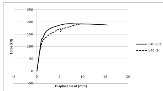
شکل (۱۲): منحنی برش پایه-تغییر مکان ستون های تسلیح شده با ۰/۳۸ درصد آرماتور CFRP و ۰/۸۵ درصد آرماتور فولادی
