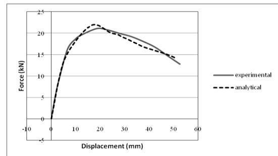
شکل (۷): منحنی برش پایه-تغییر مکان بدست آمده از نرم افزار و آزمایشگاه
