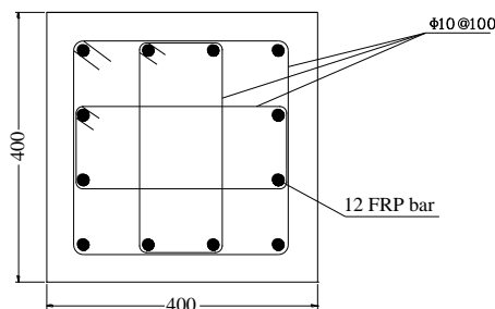
شکل (۴): جزئیات مقطع ستون‌ها (ابعاد به میلی‌متر)
