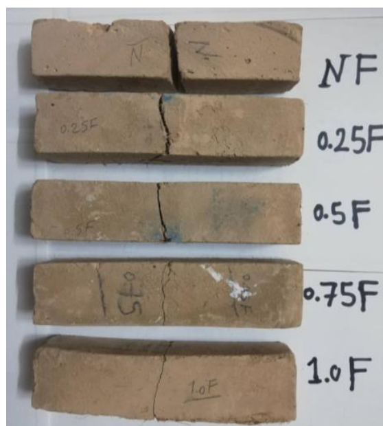
شکل ۱۴. نمونه‌ها بعد از آزمایش خمش سه نقطه‌ای
