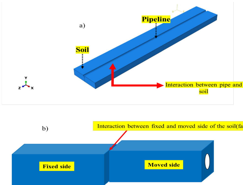
شکل ۶-الف. اندرکنش اول، میان خاک پیرامونی و لوله -ب. اندرکنش دوم، میان قطعه ثابت و متحرک خاک
