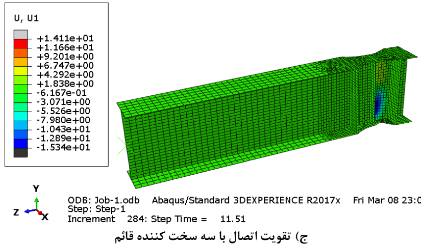
شکل ۹. تغییر شکل خارج صفحه اتصال در چرخه ششم بارگذاری در تغییر مکان نسبی ۰/۰۴۵-
