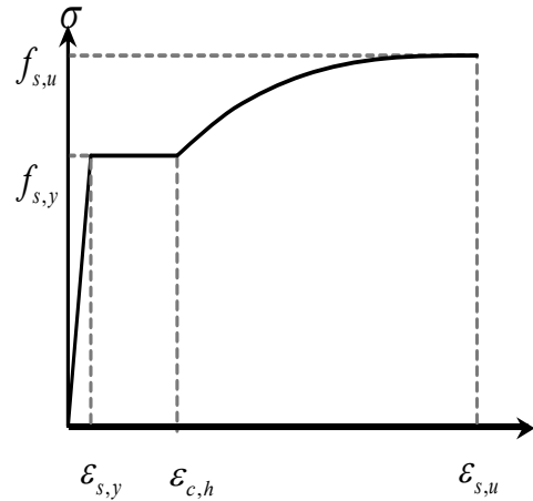
شکل ۲. مدل مواد فولاد مسلح کننده [۱۹]
