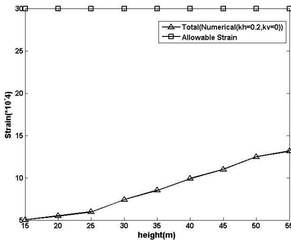
شکل ۱۵: کرنش محیطی بیشینه برای k_v=0 و k_h=0.2 با تغییر عمق
