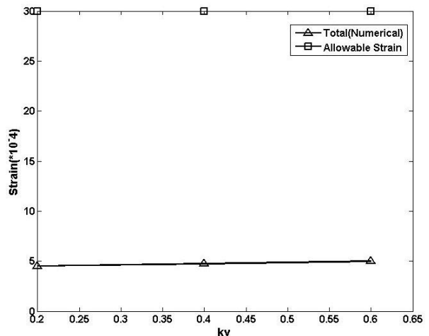
شکل ۱۳: کرنش محیطی بیشینه با مقدار ثابت k_h=0.2 در عمق ۲۰ متری
