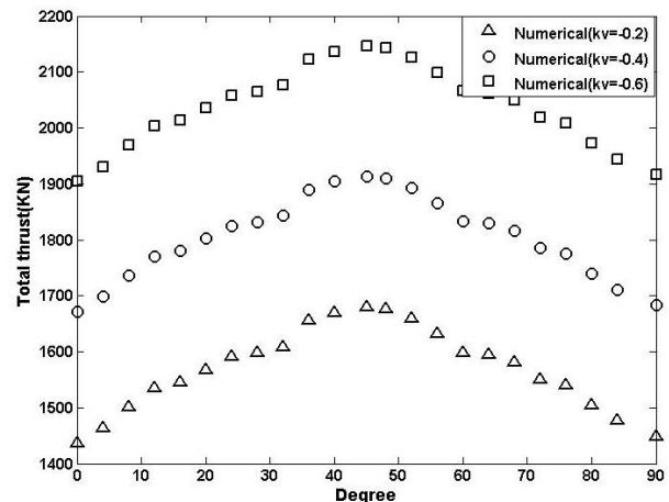
شکل ۸: توزیع نیروی محوری کل برای مقدار ثابت k_h=0.2 و مقادیر مختلف k_v در عمق ۲۰ متری
