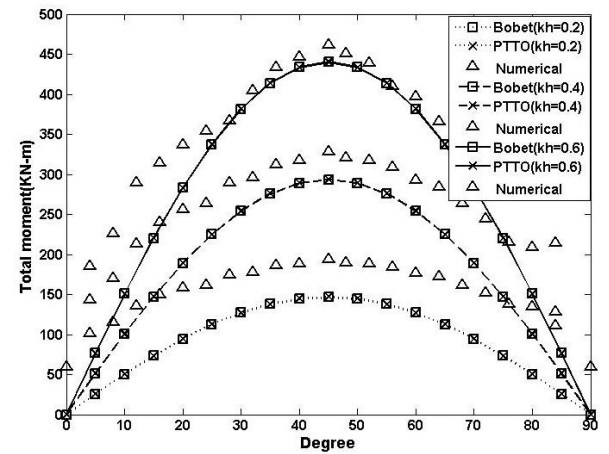
شکل ۷: توزیع لنگر خمشی کل برای مقادیر مختلف k_h در عمق ۲۰ متری
