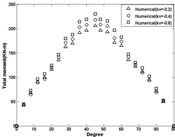
شکل ۹: توزیع لنگر خمشی کل برای مقدار ثابت k_h=0.2 و مقادیر مختلف k_v در عمق ۲۰ متری
