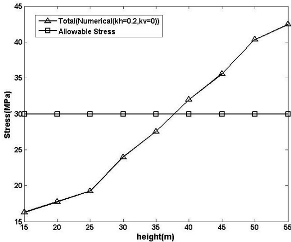
شکل ۱۴: تنش محیطی بیشینه برای k_v=0 و k_h=0.2 با تغییر عمق
