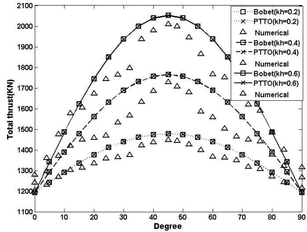
شکل ۶: توزیع نیروی محوری کل برای مقادیر مختلف k_h در عمق ۲۰ متری
