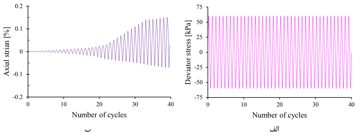
شکل ۲. نمودار تنش انحرافی (الف) و کرنش محوری (ب) در مقابل تعداد سیکلها [۲۴] Fig. 2. Deviatoric stress (a) and axial strain (b) versus of number of cycles curves
