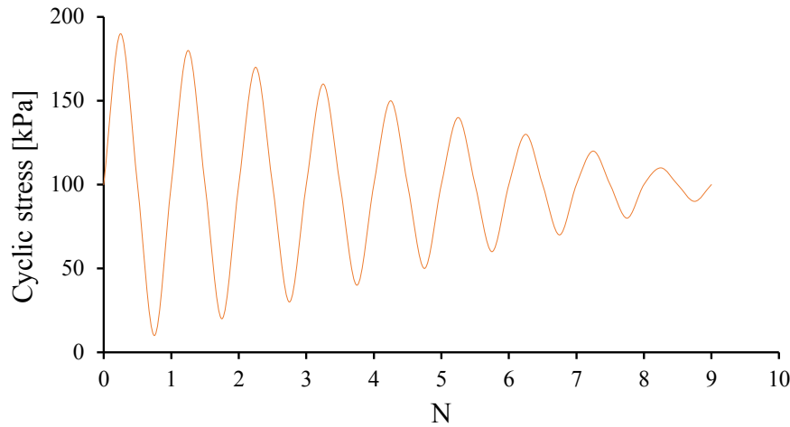
شکل ۱۶. نمونه‌های از نمودار تنش سیکلی - سیکلها (غیر یکنواخت) Fig. 16. Cyclic stress versus number of loading cycles (irregular)
