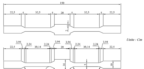
شکل (۲): اندازه‌های هسته S-BRB
