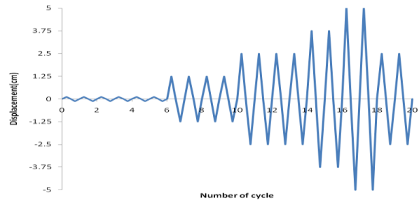
شکل (۵): پروتکل بار با \delta bm=2/5cm
