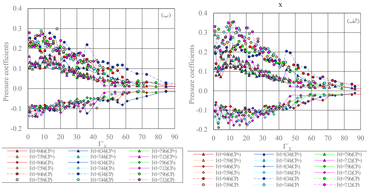
شکل ۱۰. توزیع ضرایب فشار ( C_p^+ , C_p^- و C_p ) در اعداد فرود اولیه مختلف برای حوضچه نوع دو USBR؛ (الف) S=1.00 و (ب) S=1.40 Fig. 10. Distribution of pressure coefficients ( C_p^+ , C_p^- and C_p ) in different Froude numbers for the USBR type II basin; (a) S=1.00 ; (b) S=1.40
