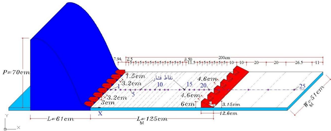
شکل ۳. آرایش نقاط فشار کف واقع در خط مرکزی حوضچه آرامش نوع دو USBR
