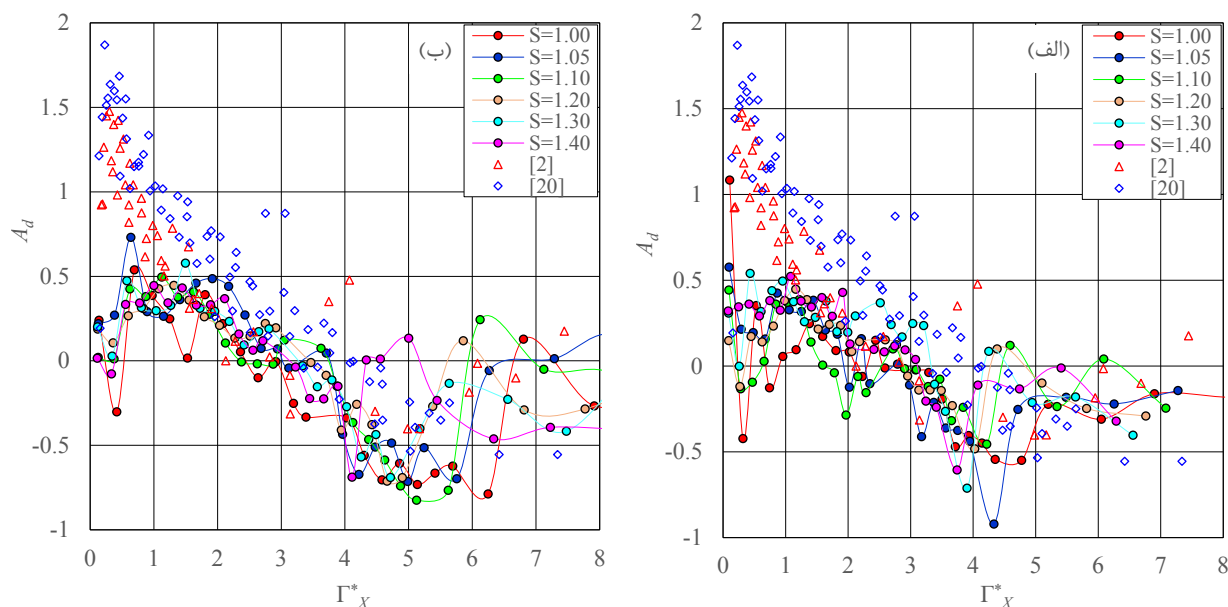
شکل ۱۳. توزیع ضریب A_d در درجه‌های استغراق مختلف برای حوضچه‌های نوع یک و دو USBR: (الف) Fr_1 = 7.12 ; (ب) Fr_1 = 9.46
