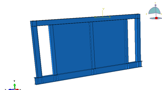
الف) مدل BESW-RMC دارای یک فرعی ستون میانی a) BESW-RMC model with one middle secondary column
