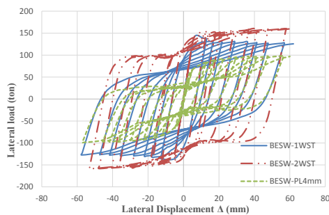
ب) منحنی های چرخه ای b) Hysteresis curves
