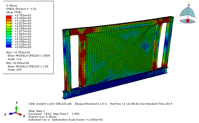
شکل ۷. کانتور تنش فون-مایسیز در انتهای بارگذاری بارافزون در مدل BESW-IPE220
