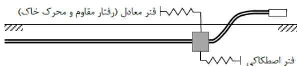
شکل ۵. نحوه ی مدل سازی اندرکنش بلوک مهار و خاک Fig. 5. Soil-block interaction modeling
