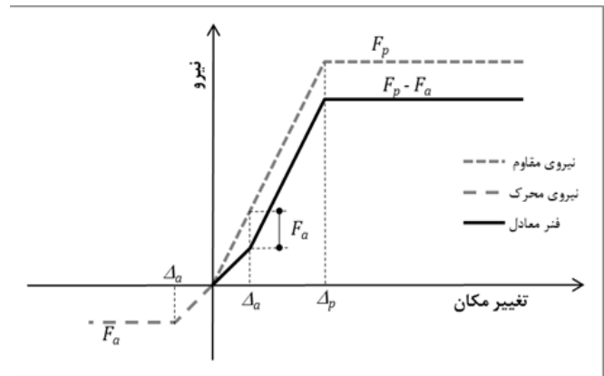
شکل ۶. نمودار نیرو-تغییر مکان فنر معادل برای مدل سازی اندرکنش خاک و بلوک
