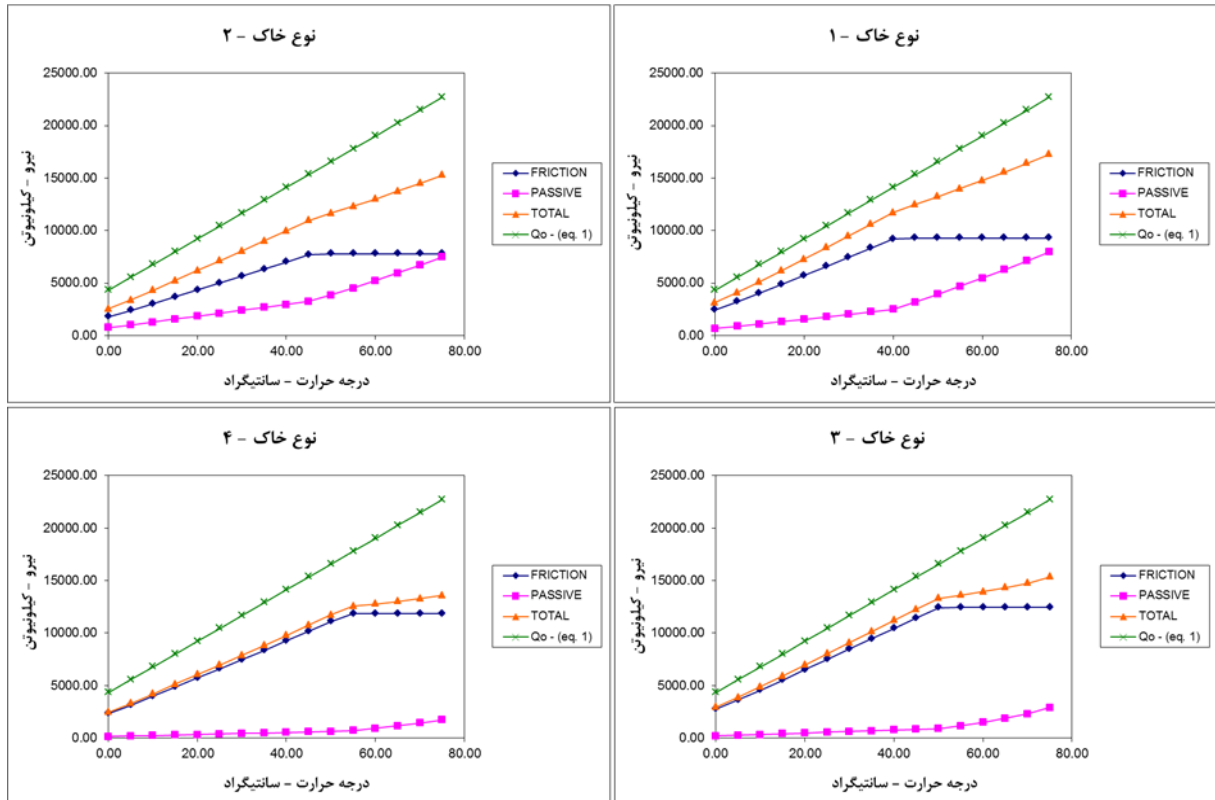
شکل ۹. نمودارهای نیروهای وارد بر بلوک مهار در درجه حرارت های مختلف برای لوله ی ۵۶ اینچ
