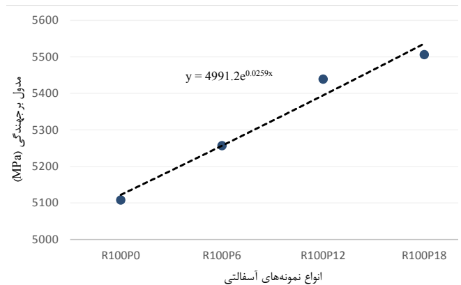
شکل ۸. نمودار نتایج مربوط به مدول برجهندگی انواع نمونه های آسفالتی حاوی ۱۰۰٪ خرده آسفالت و حاوی مقادیر مختلف پارافایبر
