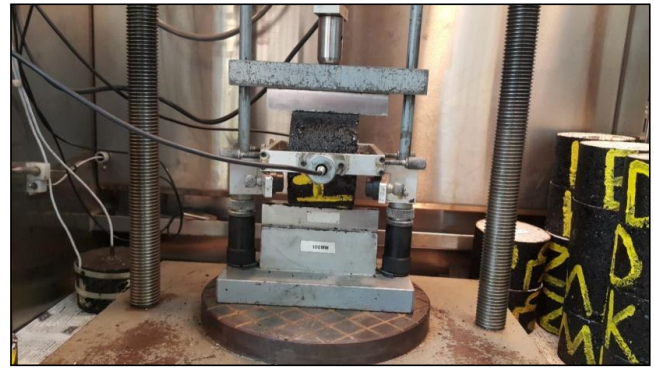
شکل ۲. تصویری از نحوه قرارگیری نمونه در آزمایش مدول برجهندگی Fig. 2. A picture of how to place a specimen in the resilient modulus test
