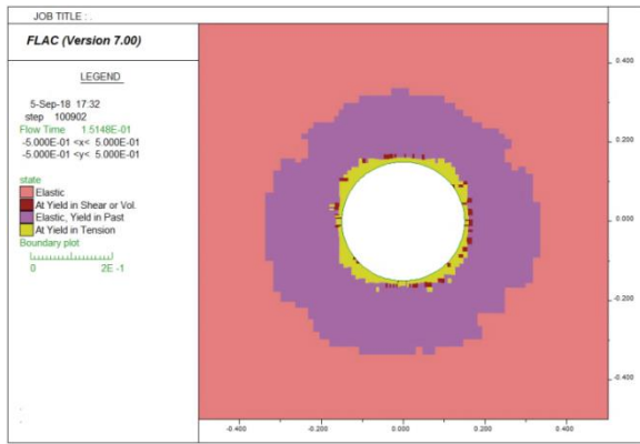
شکل ۵. وضعیت الاستوپلاستیک اطراف مدل در حفاری چاه، بدون اعمال فشار گل (چاه شماره ۱۴) Fig. 5. Elasto-plastic conditions around the model without applying mud pressure (Well No.14)
