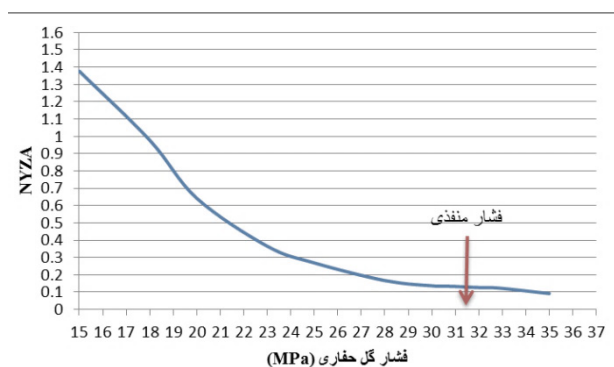
شکل ۹. میزان NYZA در فشار گل‌های مختلف در مدل‌سازی عددی (چاه شماره ۱۴) Fig. 9. NYZA at different drilling mud pressures (Well No. 14)
