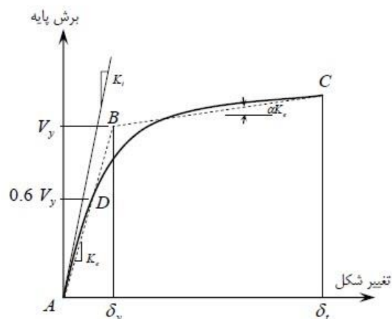
شکل ۱۶. منحنی ساده‌شده نیرو - تغییر مکان برای \alpha > 0
