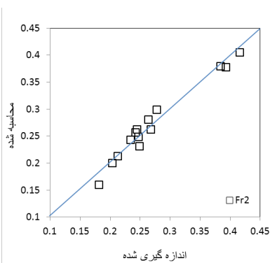
شکل ۱۳: مقایسه مقادیر محاسبه شده Fr_2 از معادله ۲۵ با مقادیر اندازه گیری شده در آزمایشگاه
