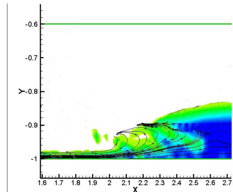
شکل ۶ خطوط جریان در محل پرش هیدرولیکی به ازای واگرایی ۲۰-۱۰ و آب پایه در X=35
