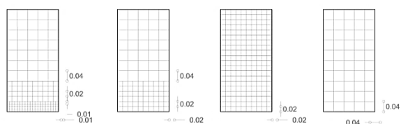
شکل ۳. انواع مش تهیه شده برای آنالیز حساسیت ابعاد مش ها (اندازه ها بر حسب متر هستند)
