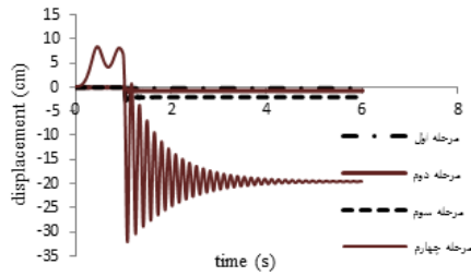
الف - تحلیل نرم افزاری
