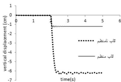
الف) قاب منظم و نامنظم ۴ دهانه
