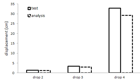
الف - جابه‌جایی قائم‌گرمه پیشینه
