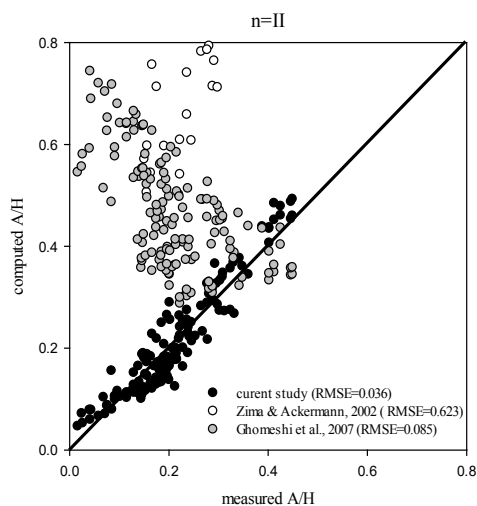
شکل ۱۲: مقایسه‌ی داده‌های آزمایشگاهی پژوهش حاضر با رابطه‌های پیشنهادی زیما و اکرم [۲]، قمشی و همکاران [۵] و رابطه ۸ این تحقیق در نوسانات مُد II
