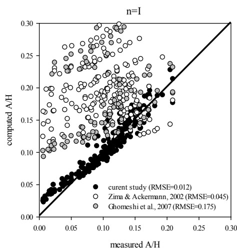
شکل ۱۱: مقایسه‌ی داده‌های آزمایشگاهی پژوهش حاضر با رابطه‌های پیشنهادی زیما و اکرم [۲] و قمشی و همکاران [۵] و رابطه ۷ این تحقیق در نوسانات مُد I
