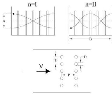
شکل ۳: شماتیک مُدهای مختلف تشکیل شده در این تحقیق
