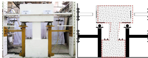
شکل ۶: دستگاه آزمایش Fig. 6. test setup
