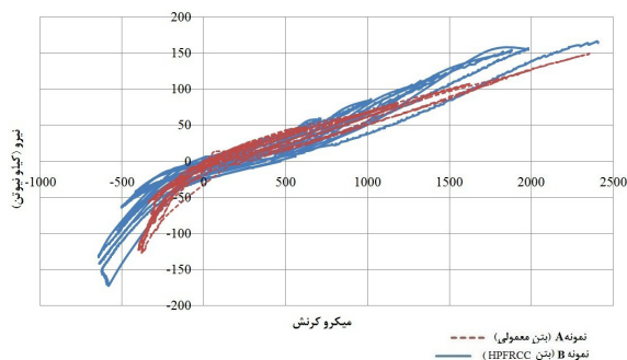
شکل ۲۲: مقایسه منحنی نیرو - کرنش آرماتور خمشی نمونه های A و B
