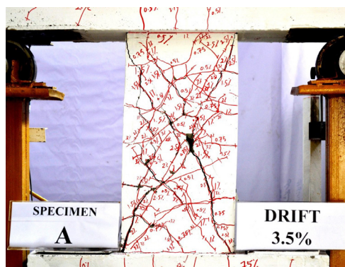
شکل ۱۲: نمونه A در انتهای بارگذاری Fig. 12. Specimen A at the end of loading
