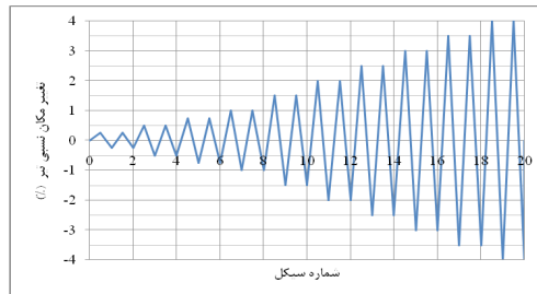
شکل ۱۰: تاریخچه بارگذاری Fig. 10. loading protocols
