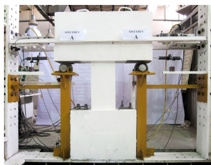
شکل ۱۱: نمونه A قبل از بارگذاری Fig. 11. Specimen A before loading
