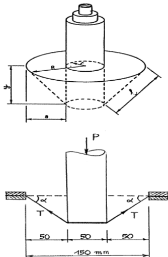
شکل (۲): انجام آزمایش سوراخ‌شدگی CBR [۱۰]
