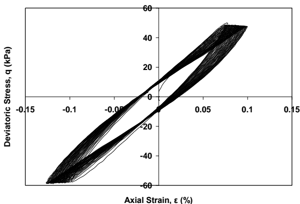
شکل (۱): منحنی‌های هیستریسیس تنش-کرنش محوری
