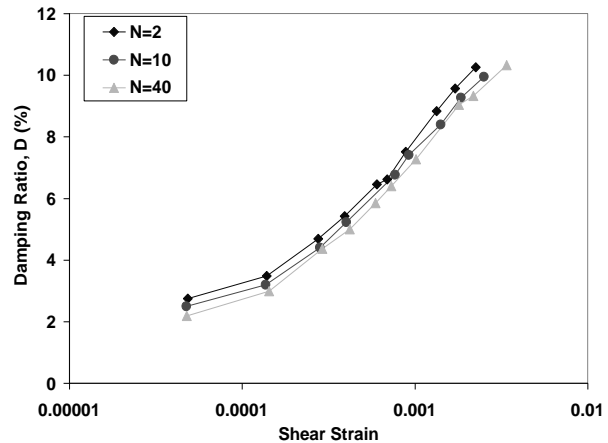
شکل (۵): تأثیر تعداد سیکلهای بارگذاری بر روی نسبت میرایی
