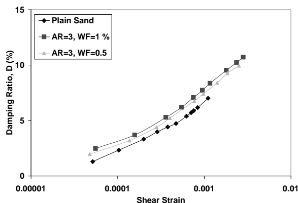
شکل (۲): تأثیر درصد وزنی الیاف بر روی نسبت میرایی نمونه های
